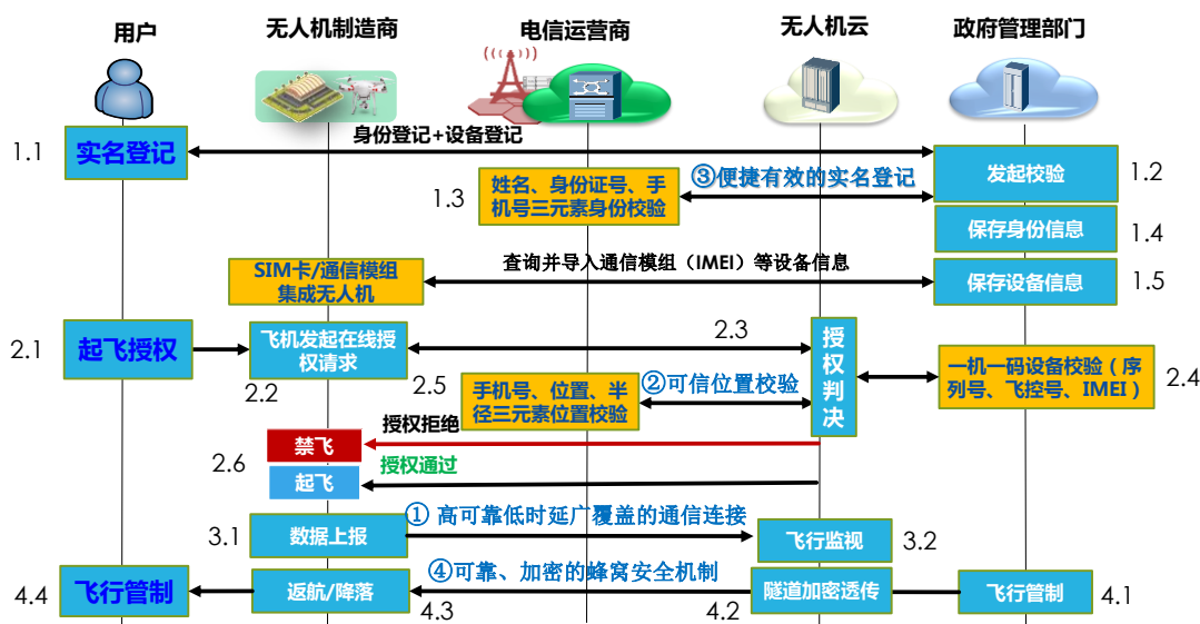
图4 联网无人机安全飞行业务流程
