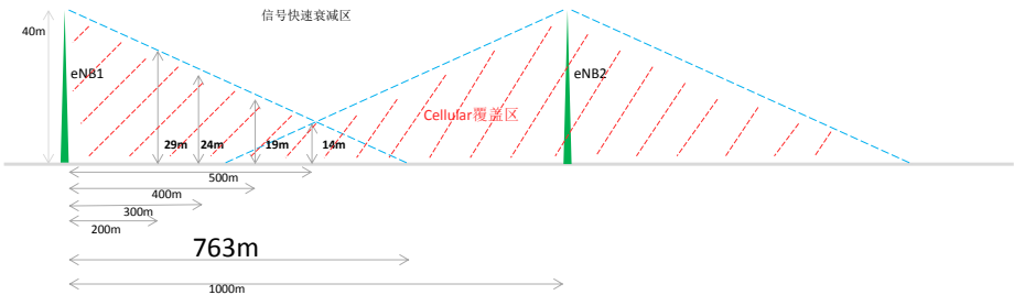
图 8 CELL_ID 粗定位精度计算
